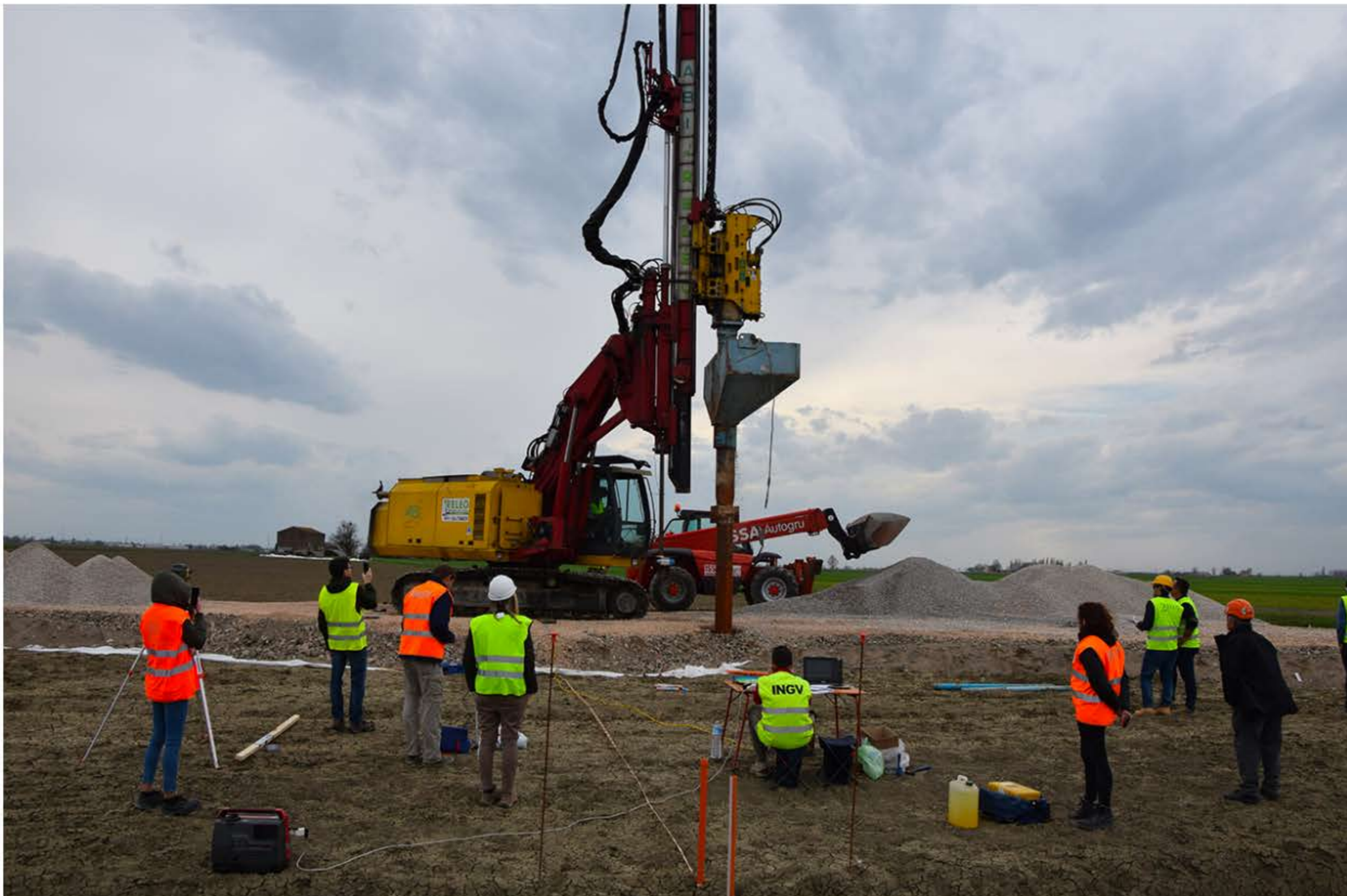
Pali in ghiaia per la riduzione del potenziale di liquefazione dei terreni. Test.
